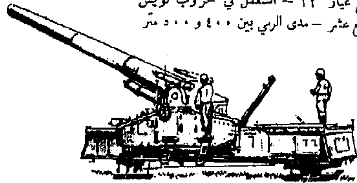
مدفع أوتوماتي عيار ٢٨٠ ميليمتراً - اختراع سنة ١٩٥٣ - المدى الأقصى للرمي : ٣٢ كم
